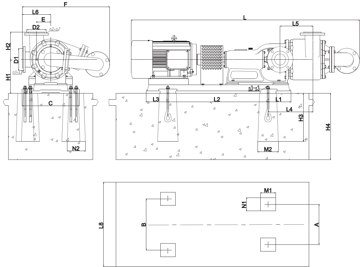
8.2 HFM-II-JS1型双级泵的外形图与安装尺寸表
