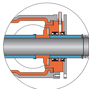
K型动力密封结构简图
