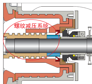
JS1新型机封结构简图
