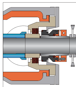
JS风冷机封结构简图
